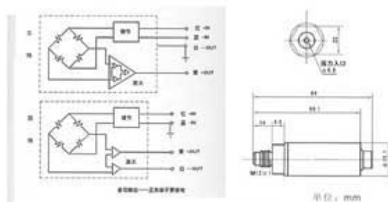
压力变送器
