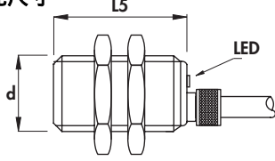
J-5形外壳尺寸
