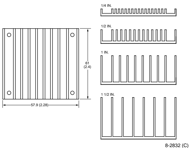
Figure 43. Longitudinal Heat Sink
