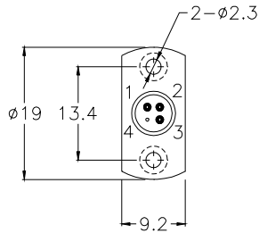
FC Receptacle T-11-155-R-SFC-AGC
