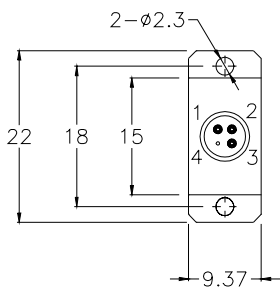
SC Receptacle T-11-155-R-SSC-AGC
