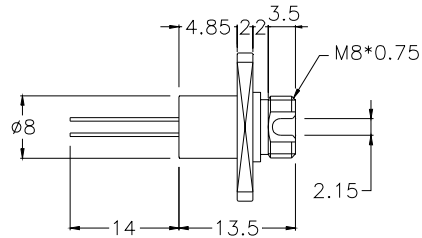
FC Receptacle T-11-155-R-SFC-AGC
