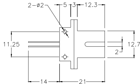
SC Receptacle T-11-155-R-SSC-AGC
