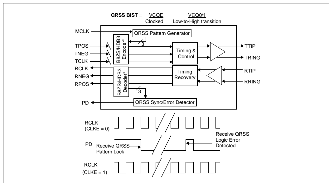
Figure 13. QRSS BIST
